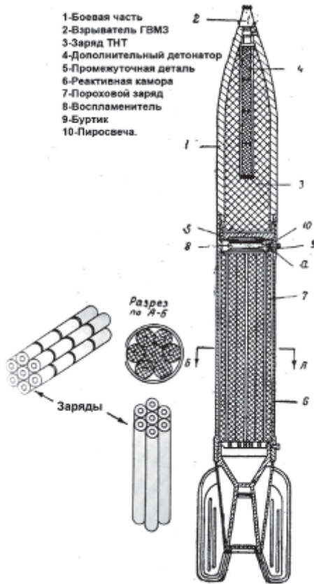
Схема реактивного снаряда М–13 для «Катюш»
